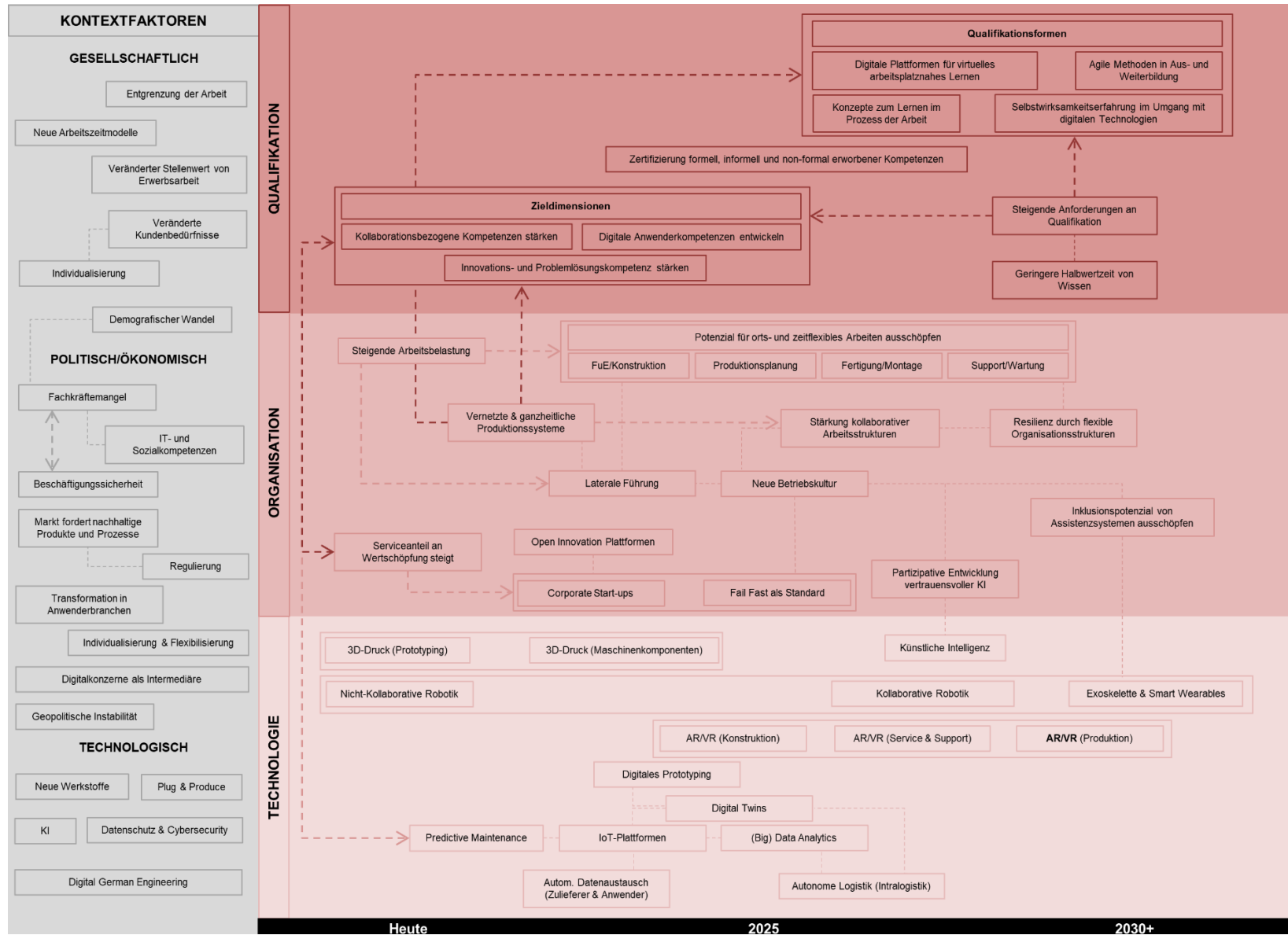
Abbildung 16: Synthetisierte Roadmap
